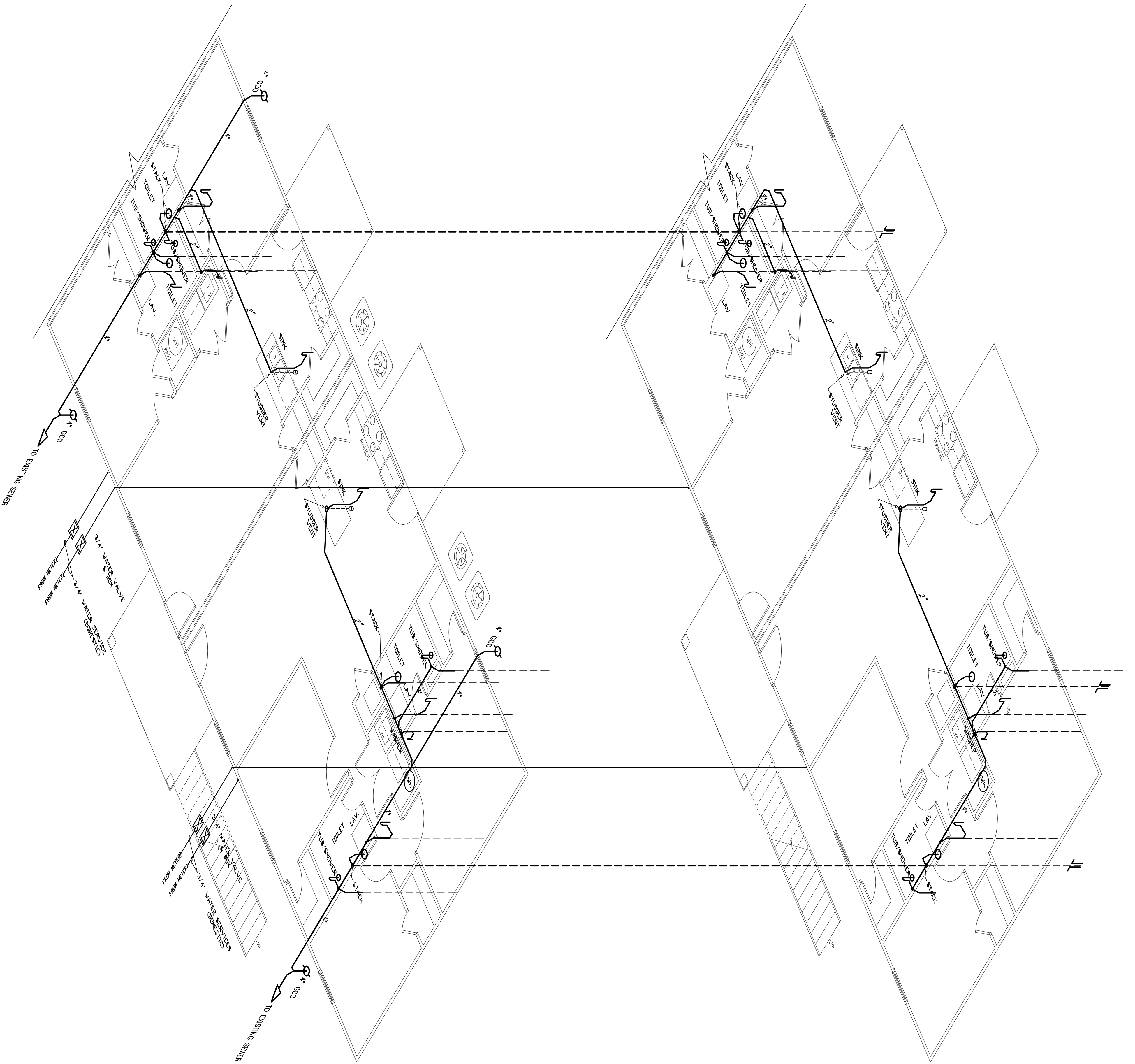
Plumbing Riser Diagram Scale: 1/4" = 1'-0"
